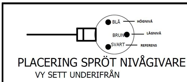
Bild 2: Nivågivare sett underifrån
