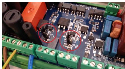
Bild 14 Fasta kortet där byglarna är inringade i rött
