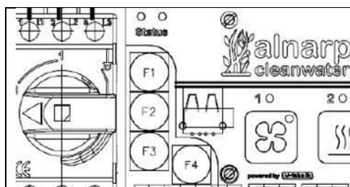
Bild 9: Säkringar
