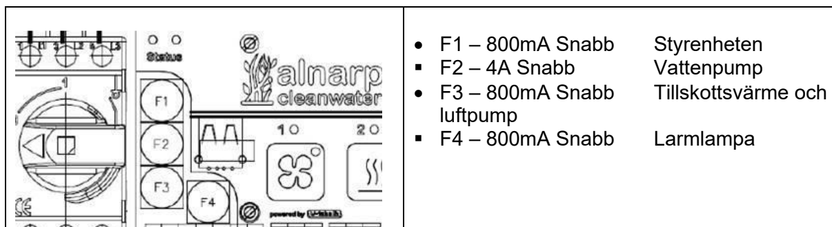
Bild 9: Säkringar
