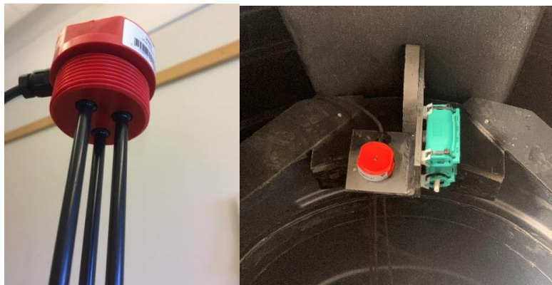
Bild 7: Nivågivare
